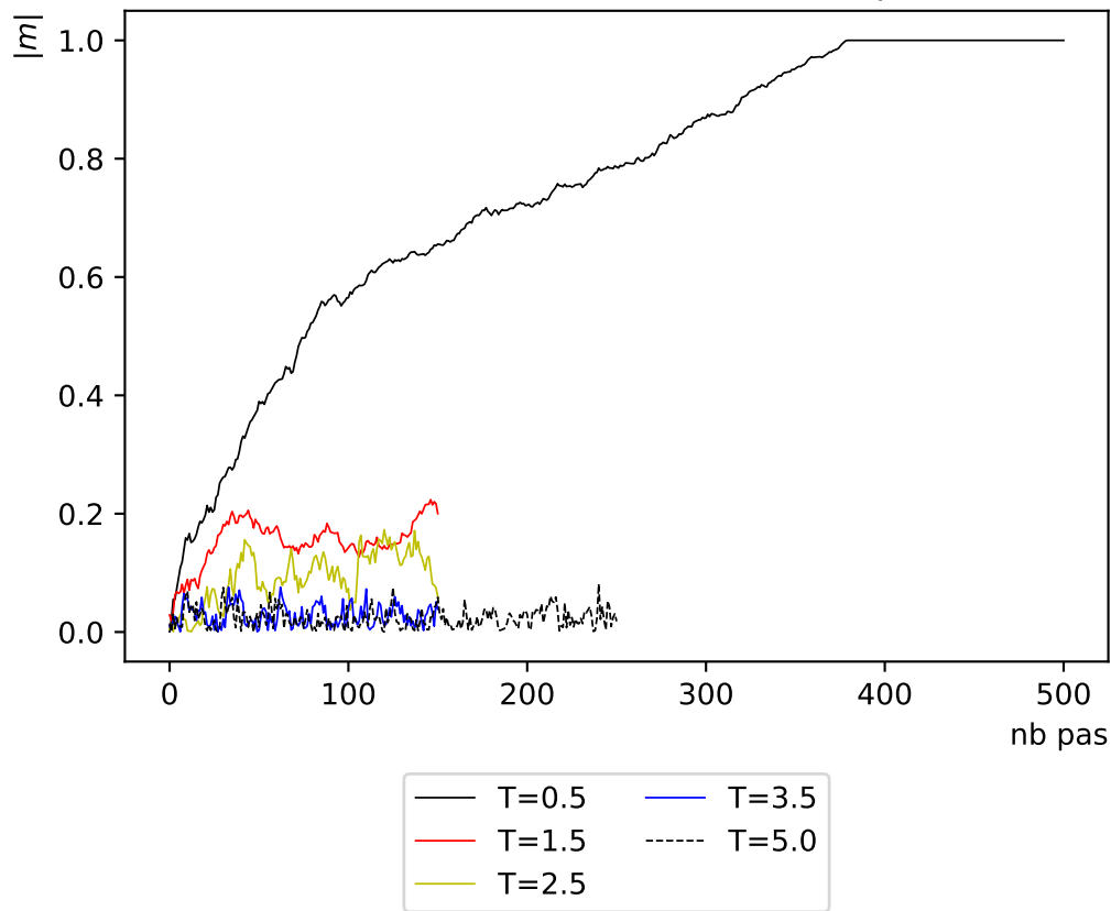
Evolution de l'aimantation sur critère Estimation par intervalle, N=64
